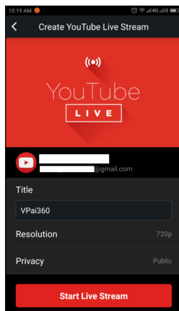
Figura 6: Interfaz registrada
