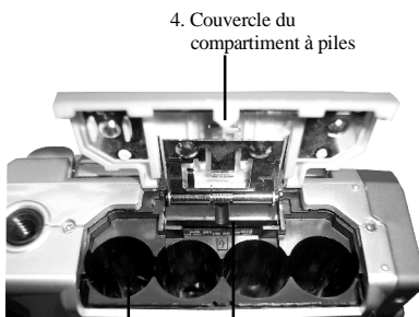
2. Compartiment à piles 3. Fente pour Carte mémoire/commutateur multimédia 4. Couvercle du compartiment à piles
